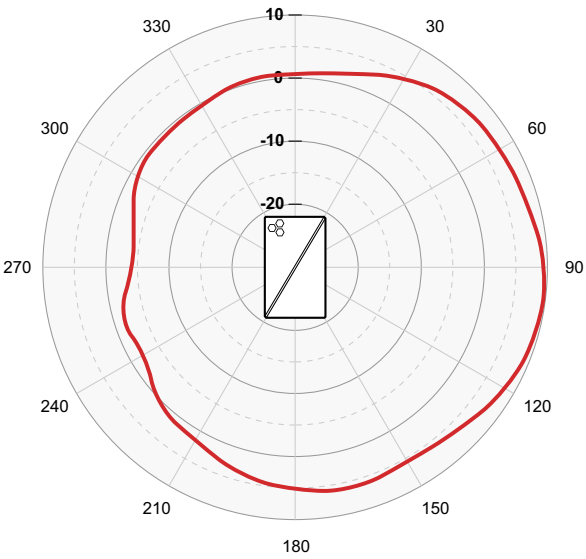
Azymut - 5 GHz
