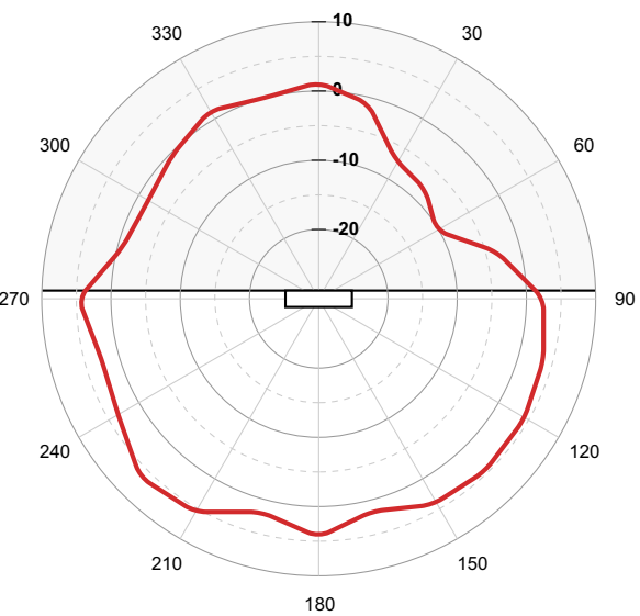
Wysokość - 2.4 GHz
