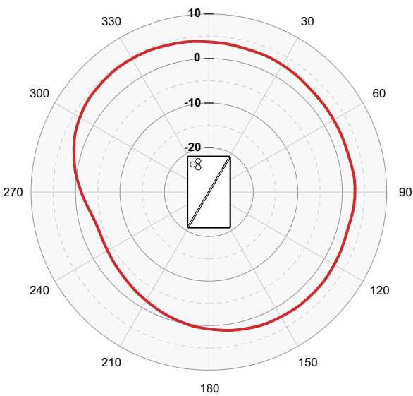
Azymut - 2.4 GHz
