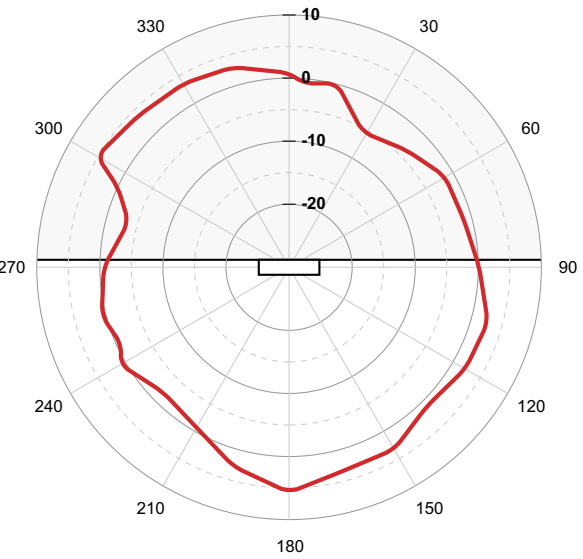
Wysokość - 5 GHz
